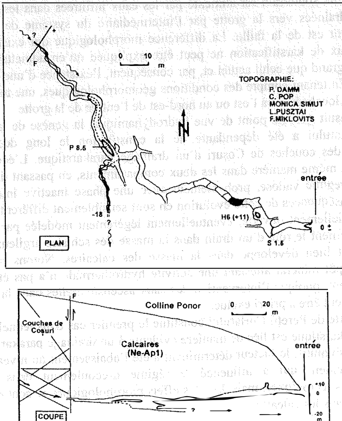
Fig.2. - La Grotte de Pereții Corlatului, plan et coupe.
